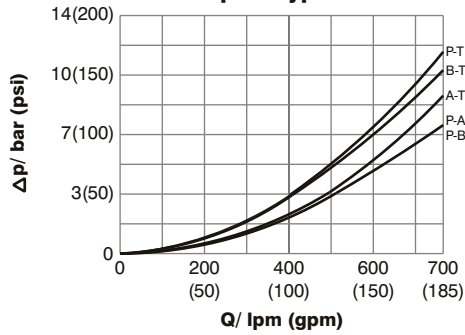
Spool Type 02
