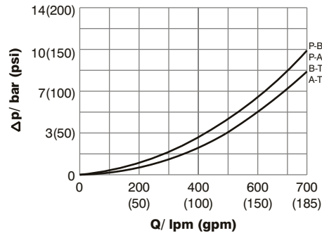
Spool Type 11
