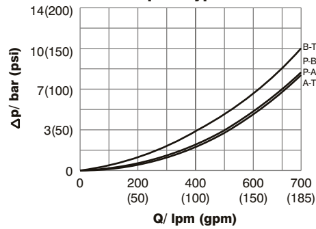
Spool Type 09
