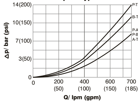
Spool Type 08
