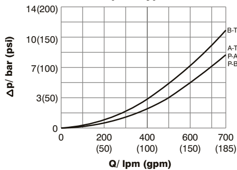
Spool Type 03
