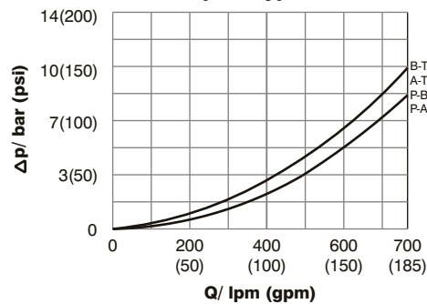
Spool Type 11
