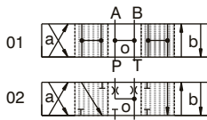
Spool Type 01
